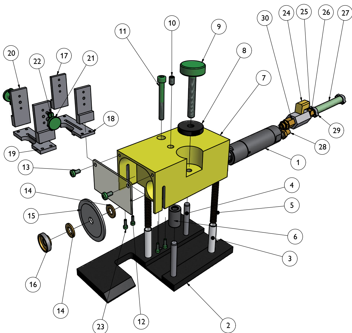
Abb. 3: Explosionszeichnung
