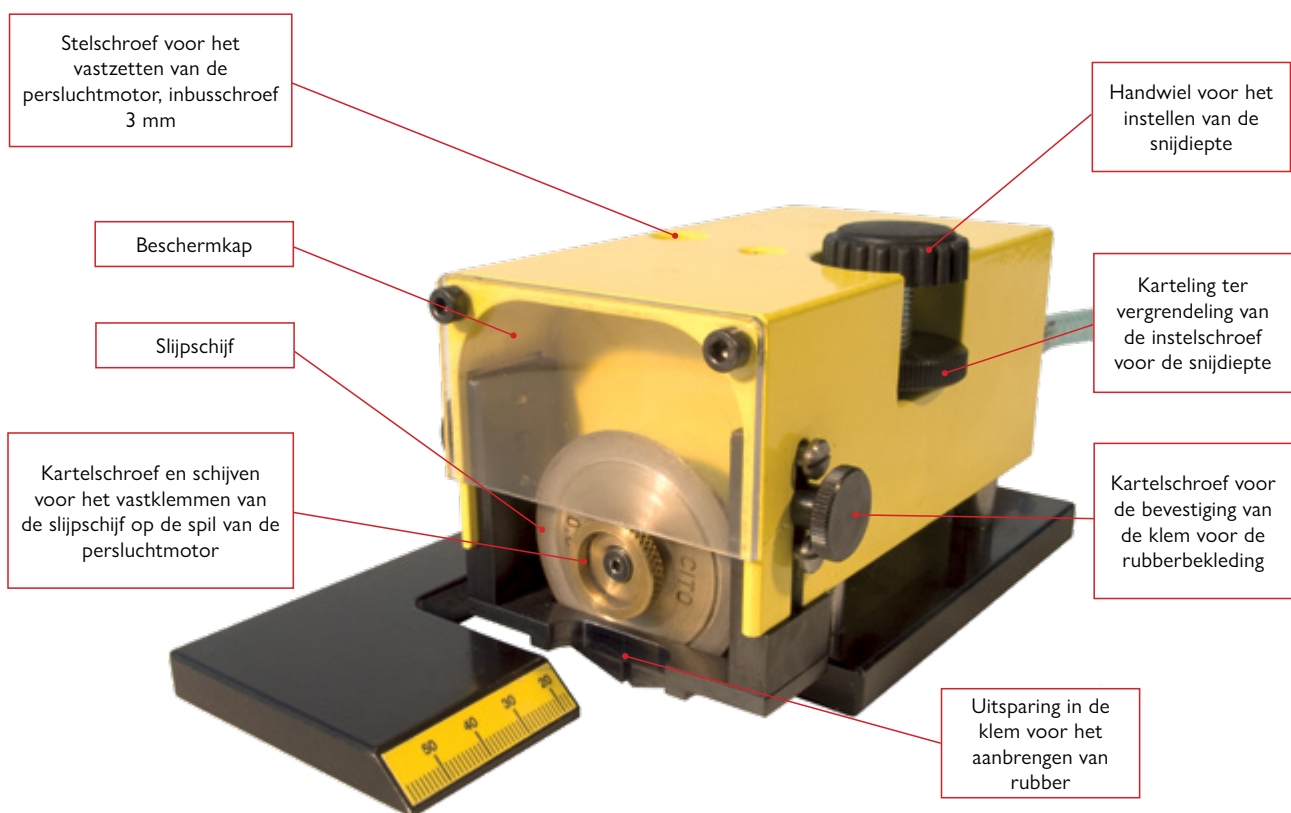
Afb. 2: CG3-bedieningselementen
