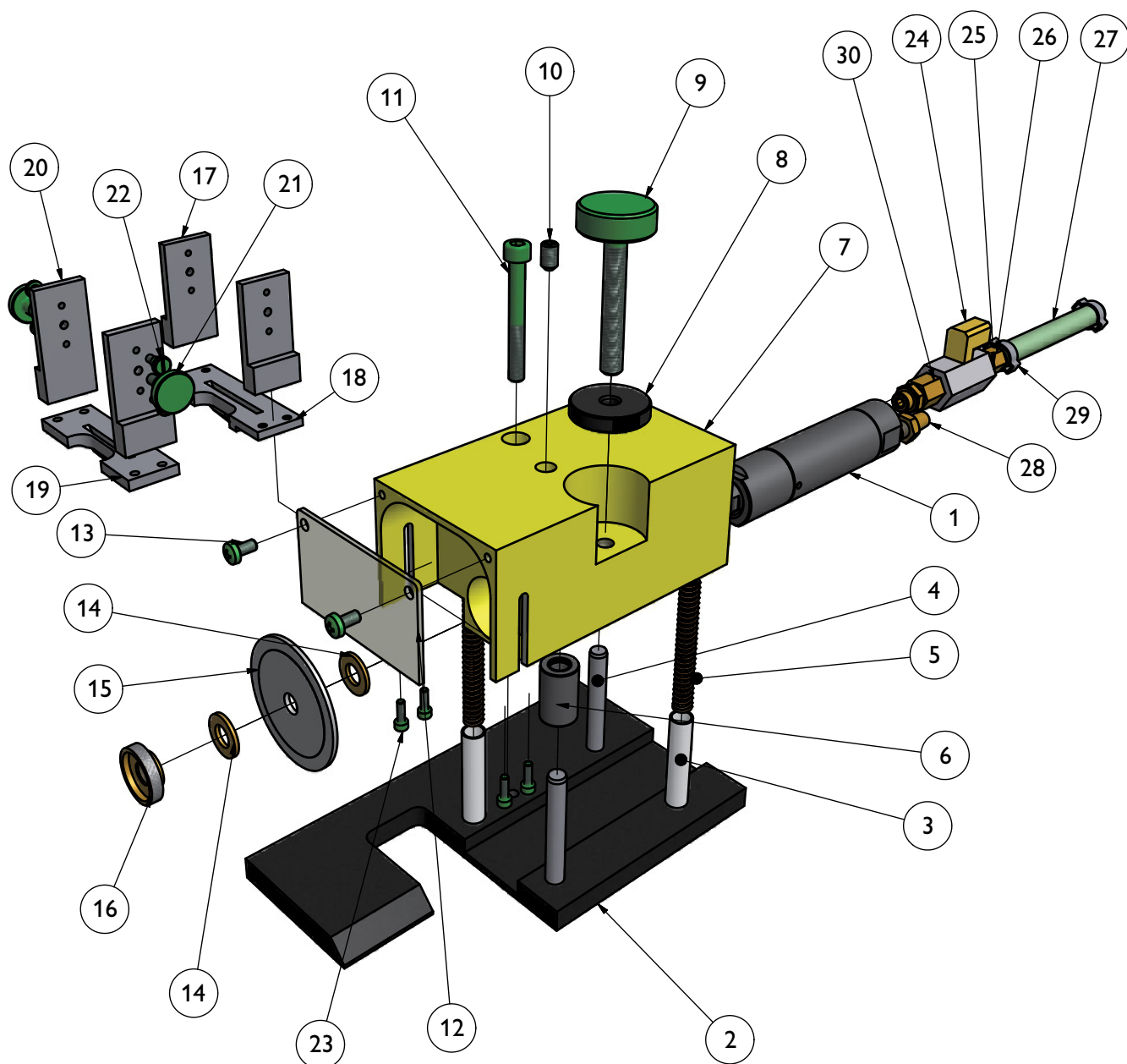
Afb. 3: Explosietekening
